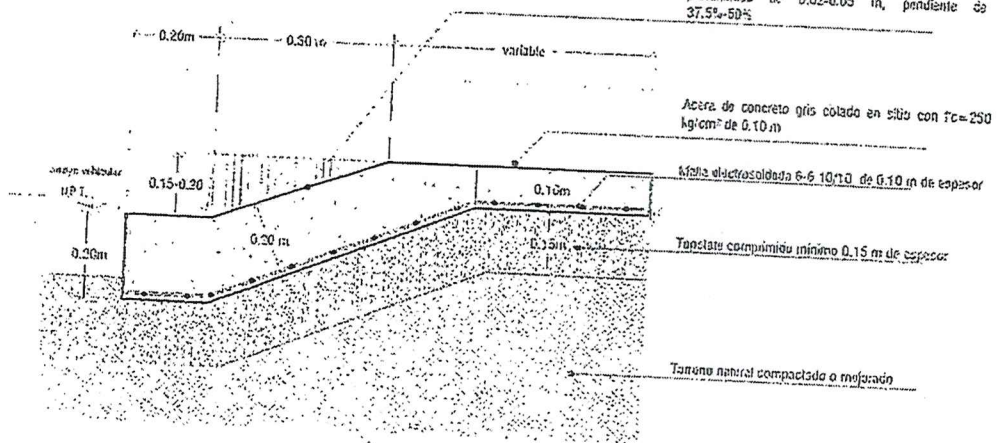
DET. Rampa en accesos vehiculares corte a-a'
